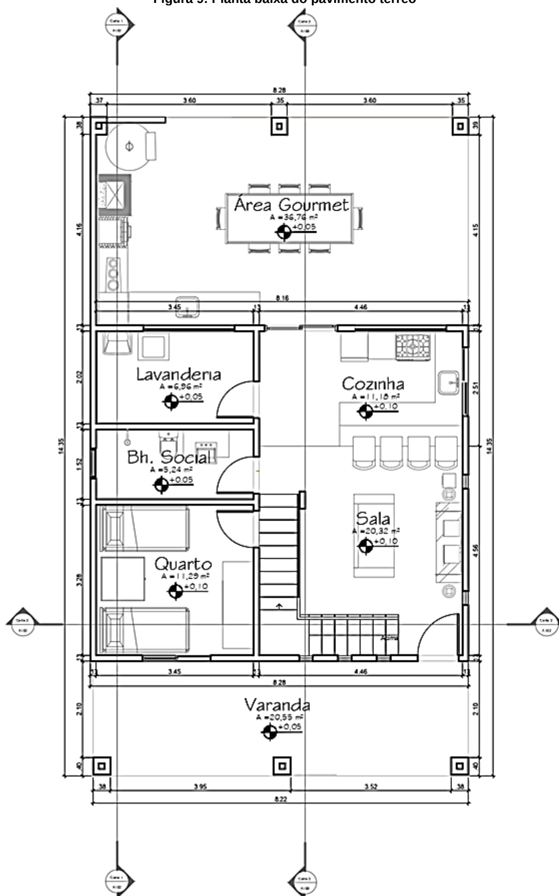
Figura 9: Planta baixa do pavimento térreo
