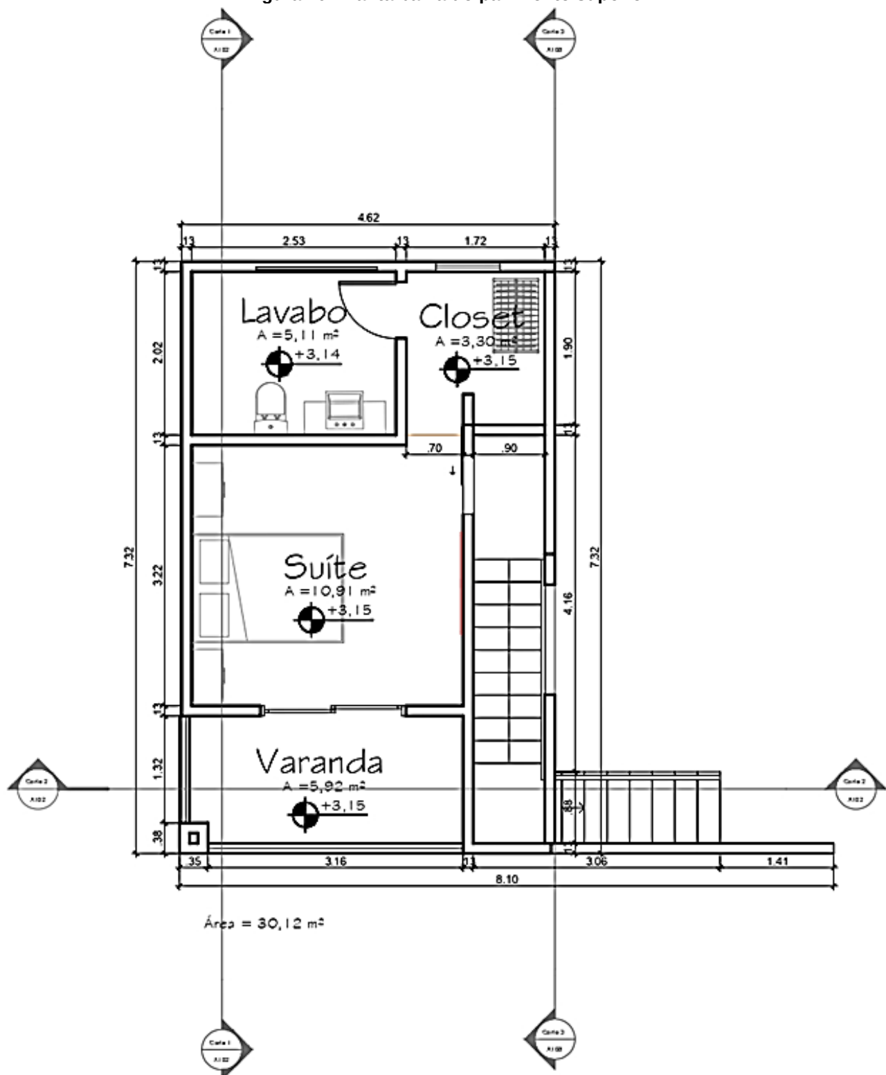
Figura 10: Planta baixa do pavimento superior
