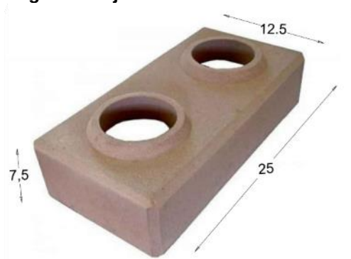
Figura 7: Tijolo modular solo-cimento
