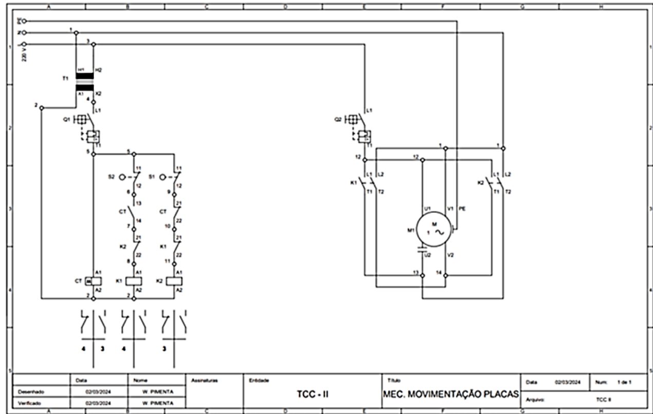
Figura 5 - Planta representativa do desenho do MAF (Mecanismo de Abertura e Fechamento) representada em apêndice
