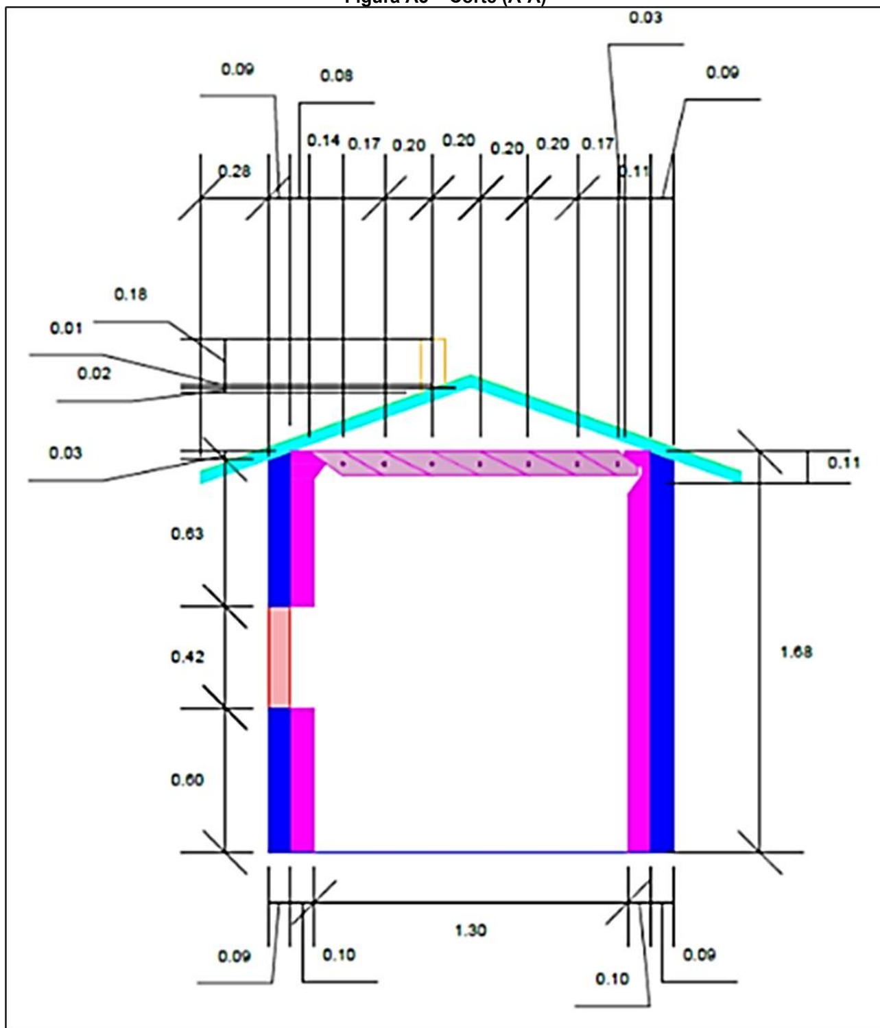
Figura A5 – Corte (A-A)
