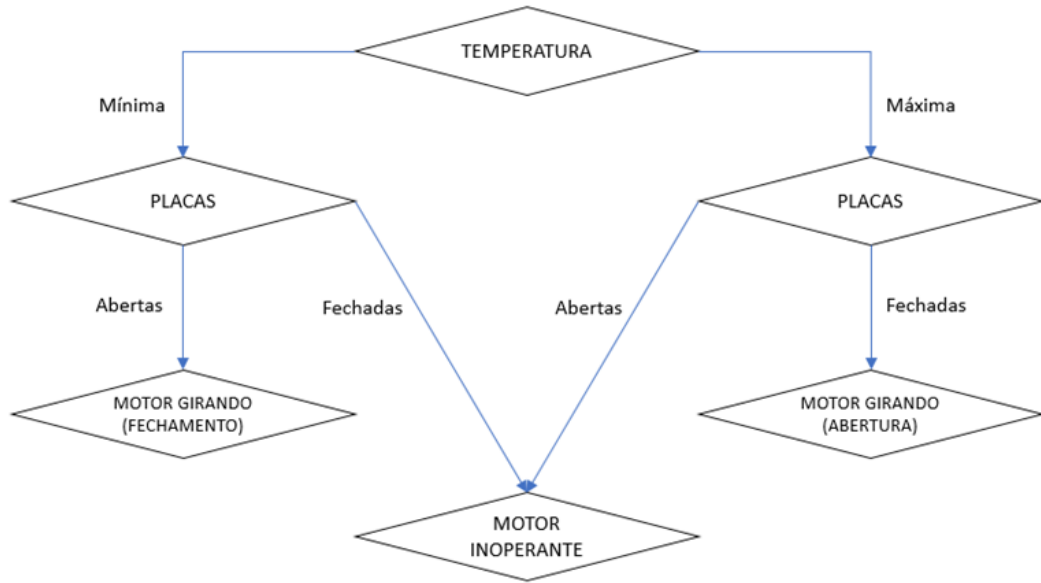
Figura 6 – Algoritmo de funcionamento do Mecanismo de Abertura e Fechamento das placas de XPS
