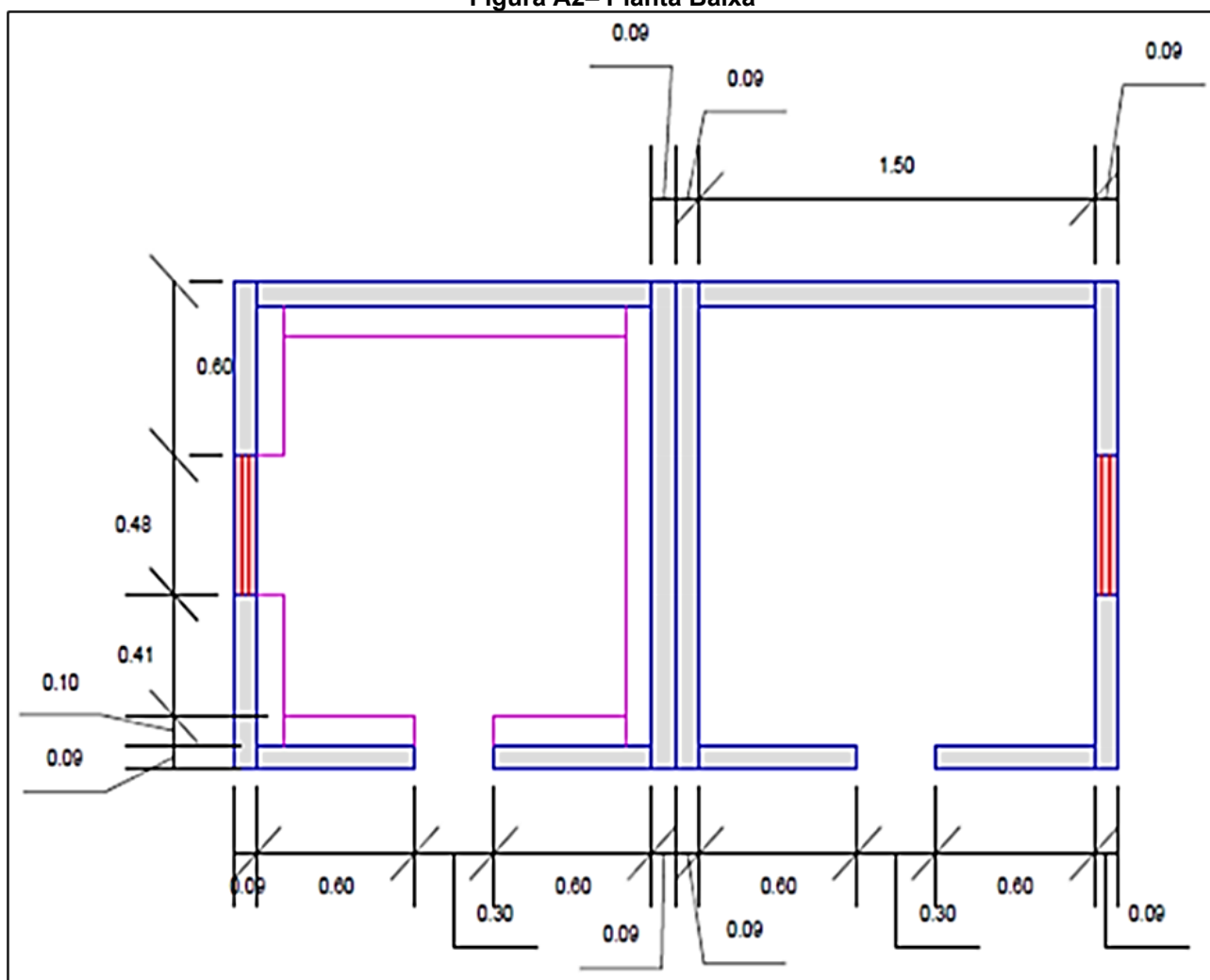
Figura A2– Planta Baixa
