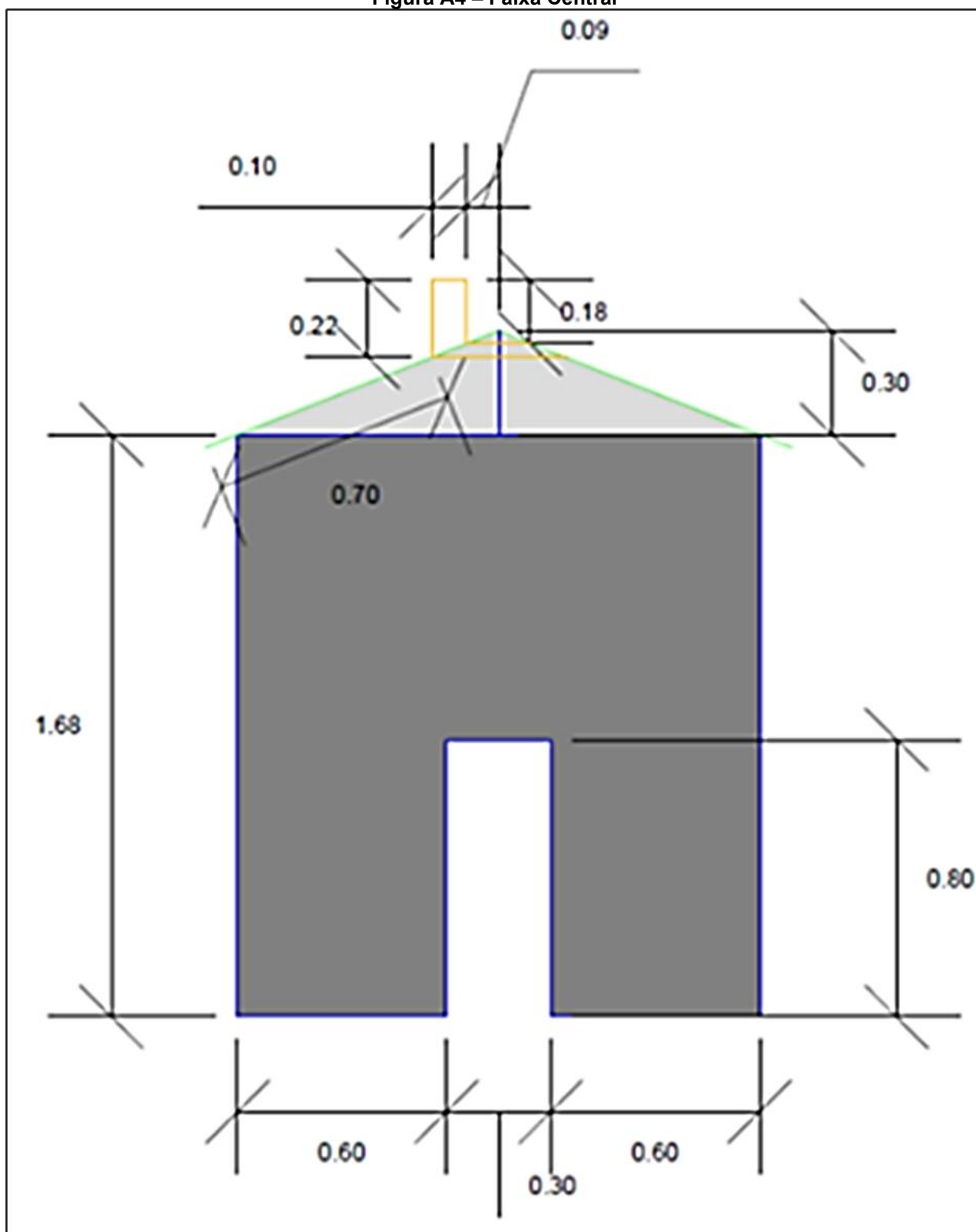
Figura A4 – Faixa Central
