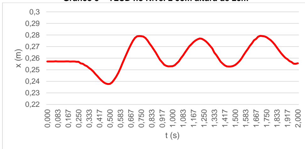
Gráfico 5 – TLCD no Nível 2 com altura de 2cm
