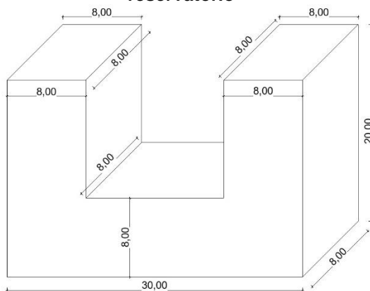
Figura 13 – Projeto para confecção do reservatório
