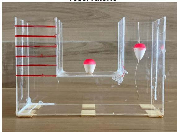
Figura 14 – Projeto para confecção do reservatório
