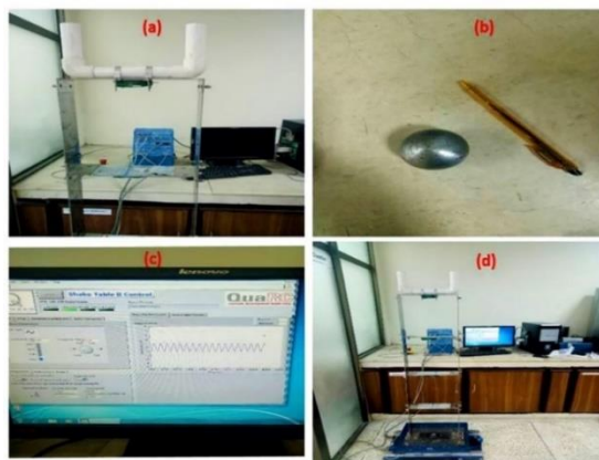
Figura 6 – (a) modelo TLCBD; (b) Esfera de aço esférica; (c) janela do software QuaRC; (d) Toda a configuração experimental
