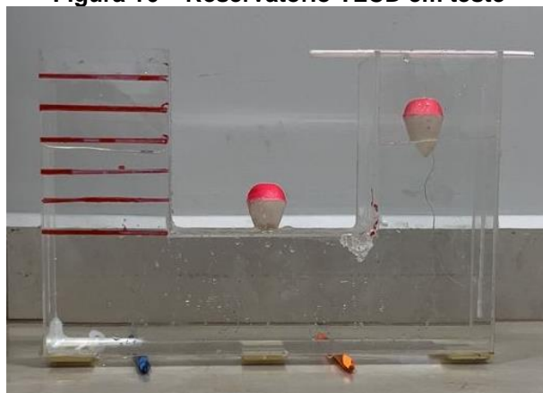
Figura 16 – Reservatório TLCD em teste
