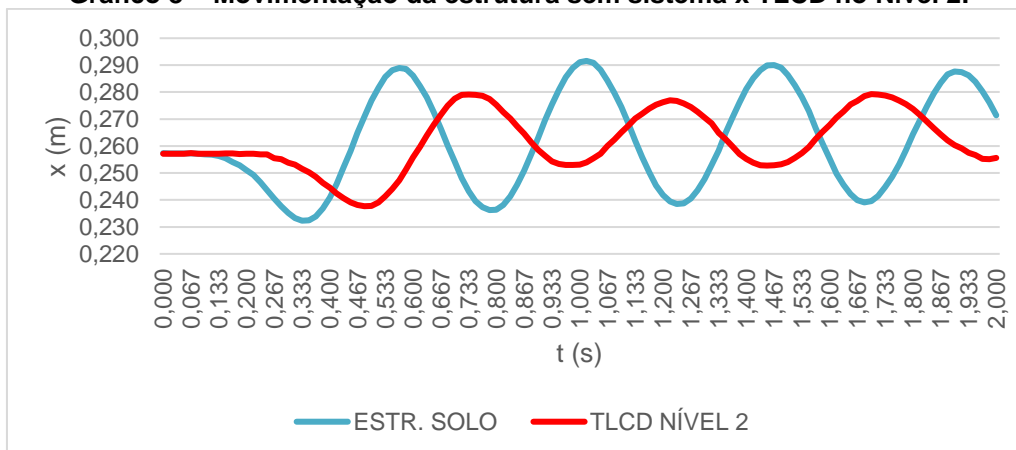
Gráfico 8 – Movimentação da estrutura sem sistema x TLCD no Nível 2.
