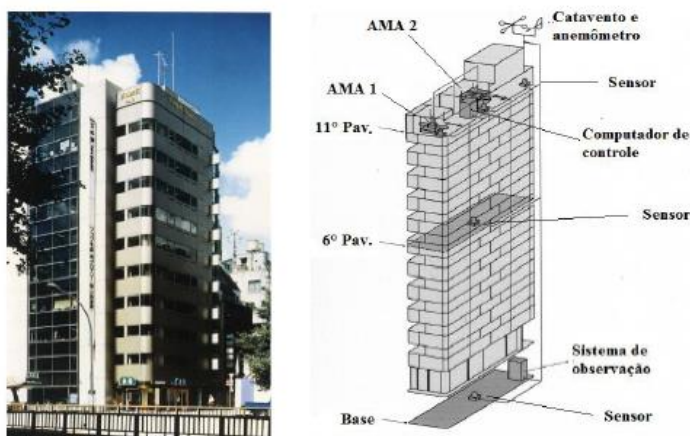
Figura 3 - Sistema de controle ativo: à esquerda o Edifício Kyobashi-Seiwa e à direita uma ilustração do sistema de controle
