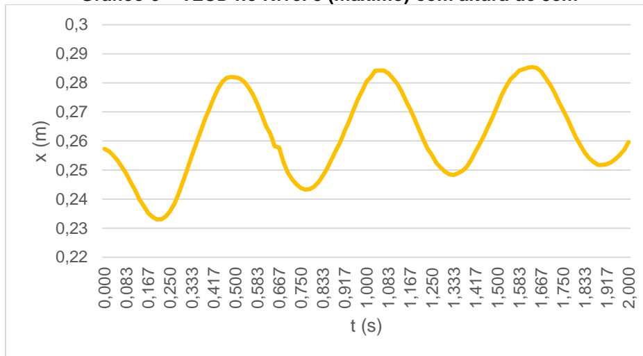
Gráfico 6 – TLCD no Nível 5 (máximo) com altura de 8cm
