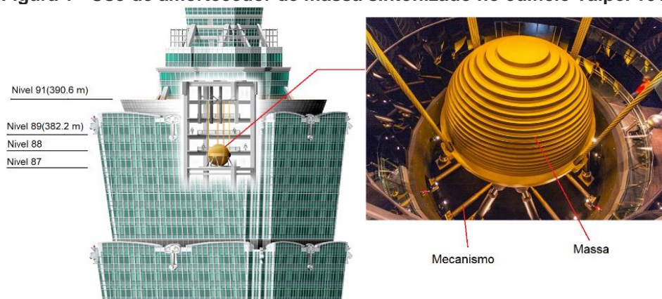
Figura 1 - Uso de amortecedor de massa sintonizado no edifício Taipei 101.
