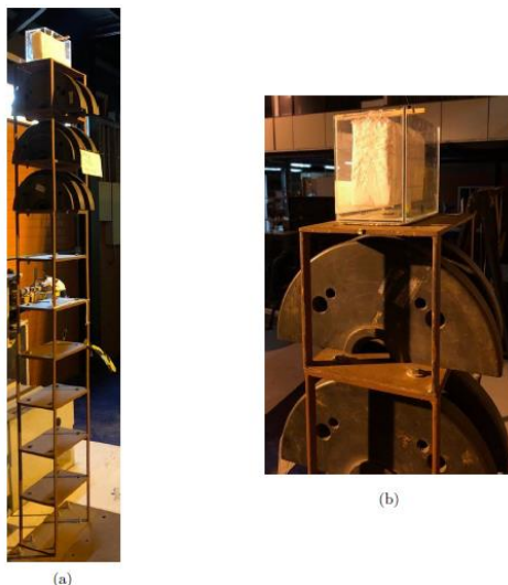
Figura 9 – Sistema acoplado: (a) vista geral do sistema e (b) detalhe da posição do ACLS
