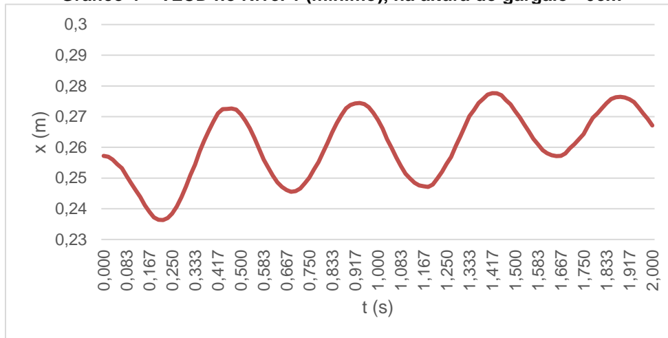
Gráfico 4 – TLCD no Nível 1 (mínimo), na altura do gargalo - 0cm
