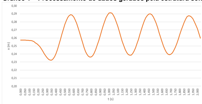
Gráfico 1 – Processamento de dados gerados pela estrutura solo
