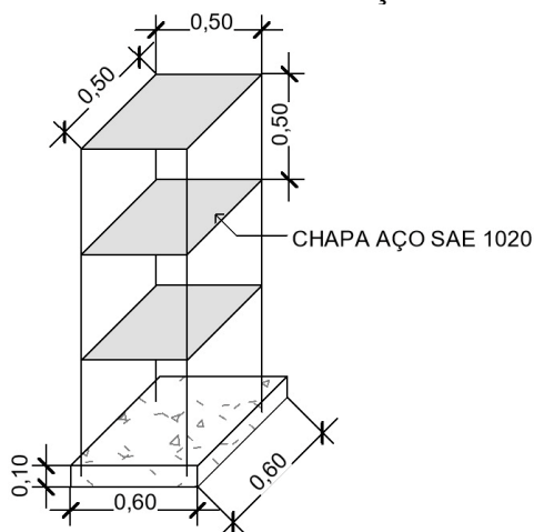
Figura 11 – Projeto para confecção da estrutura da edificação
