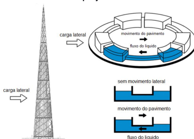
Figura 2 - Uso de amortecedor de líquido sintonizado no projeto Millenium Tower
