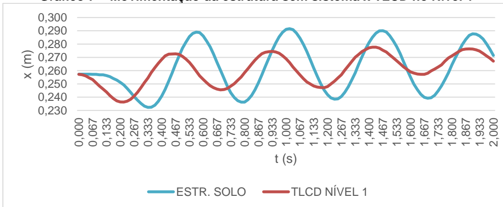
Gráfico 7 – Movimentação da estrutura sem sistema x TLCD no Nível 1
