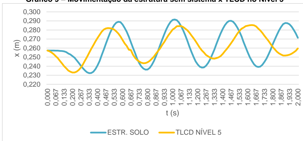
Gráfico 9 – Movimentação da estrutura sem sistema x TLCD no Nível 5
