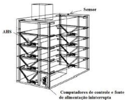
Figura 4 – Sistema de controle semiativo: à esquerda o Edifício Kajima Shizuoka e à direita ilustração do respectivo sistema de controle
