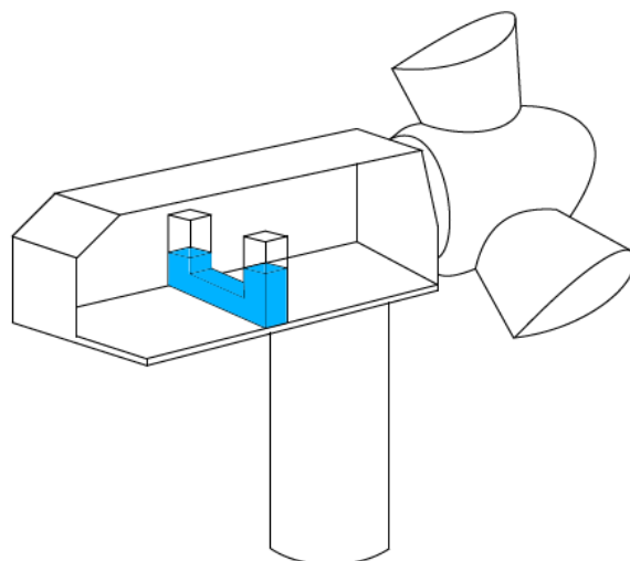
Figura 8 – Exemplo de um TLCD em uma turbina eólica
